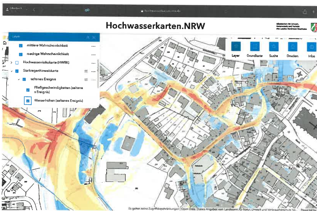
Seltenes Starkregenereignis: Wasserhöhen und Fließgeschwindigkeiten
