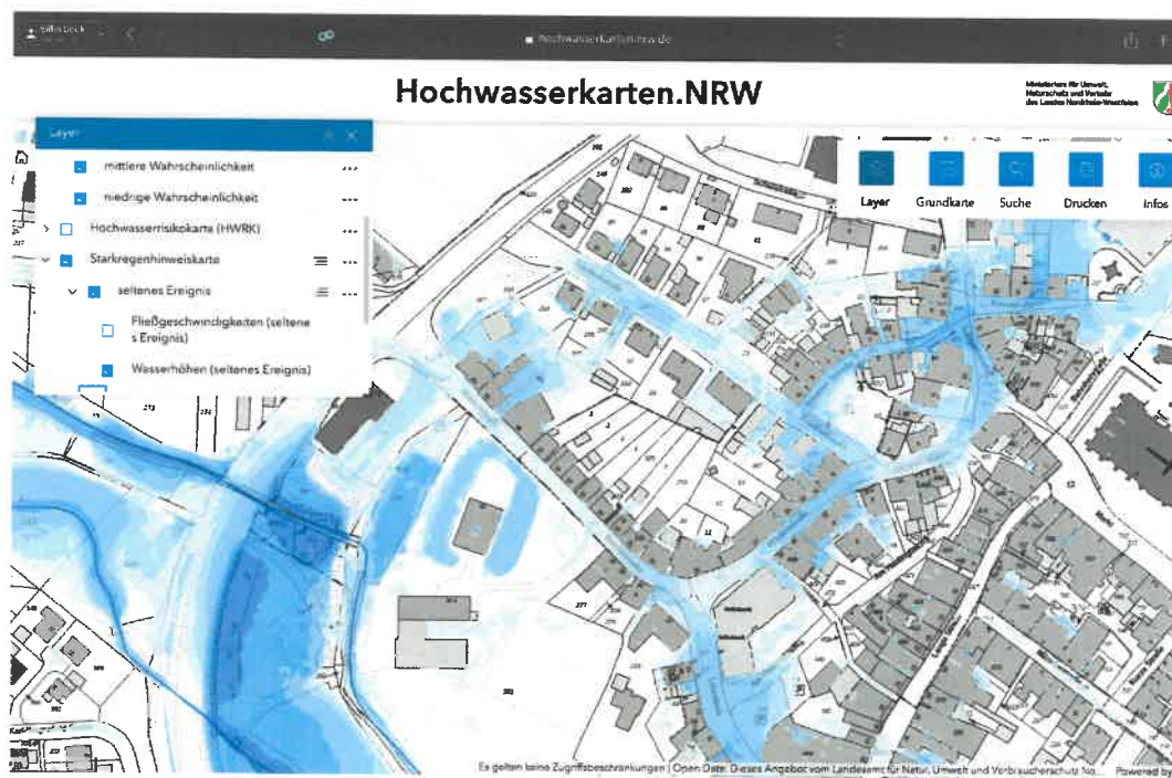
Seltenes Starkregenereignis: Wasserhöhen
