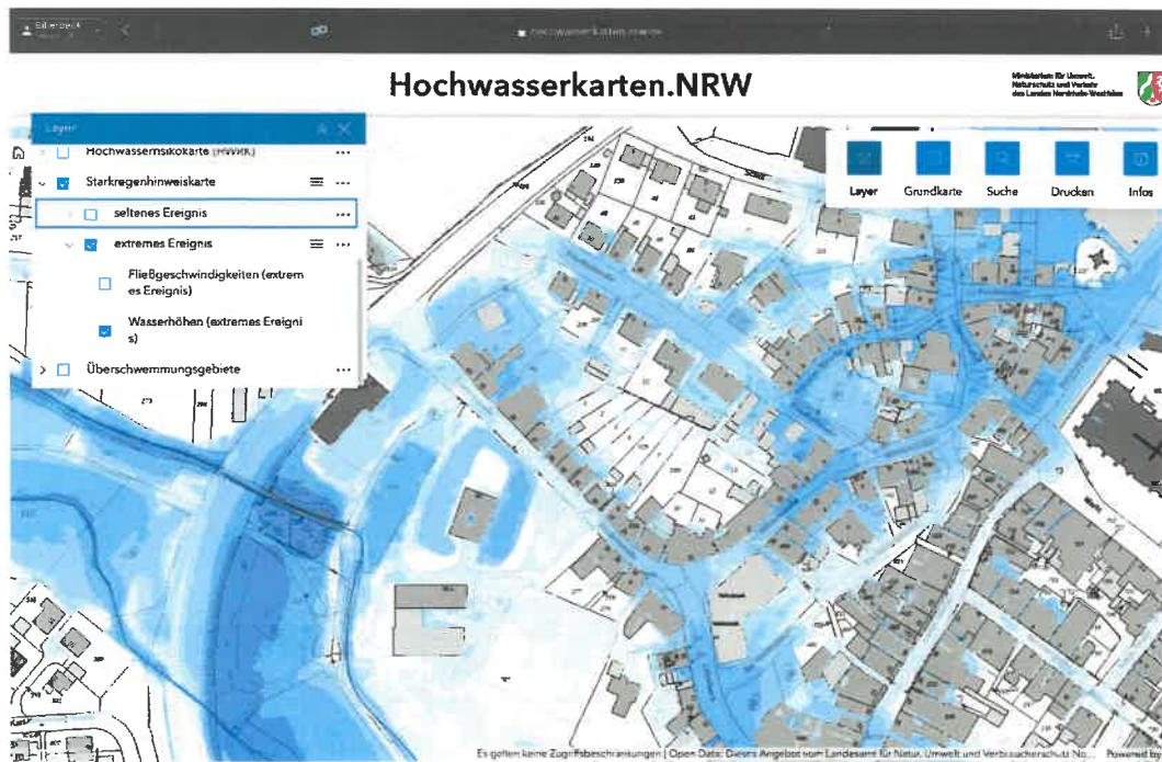
Extremes Starkregenereignis: Wasserhöhen
