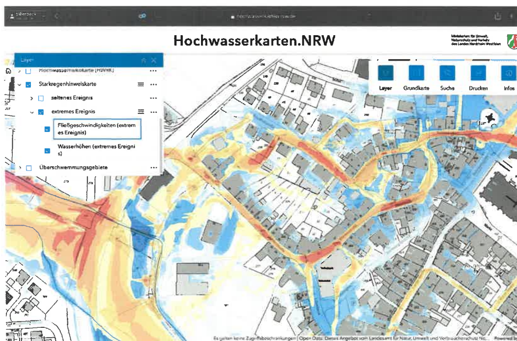
Extremes Starkregenereignis: Wasserhöhen und Fließgeschwindigkeiten
