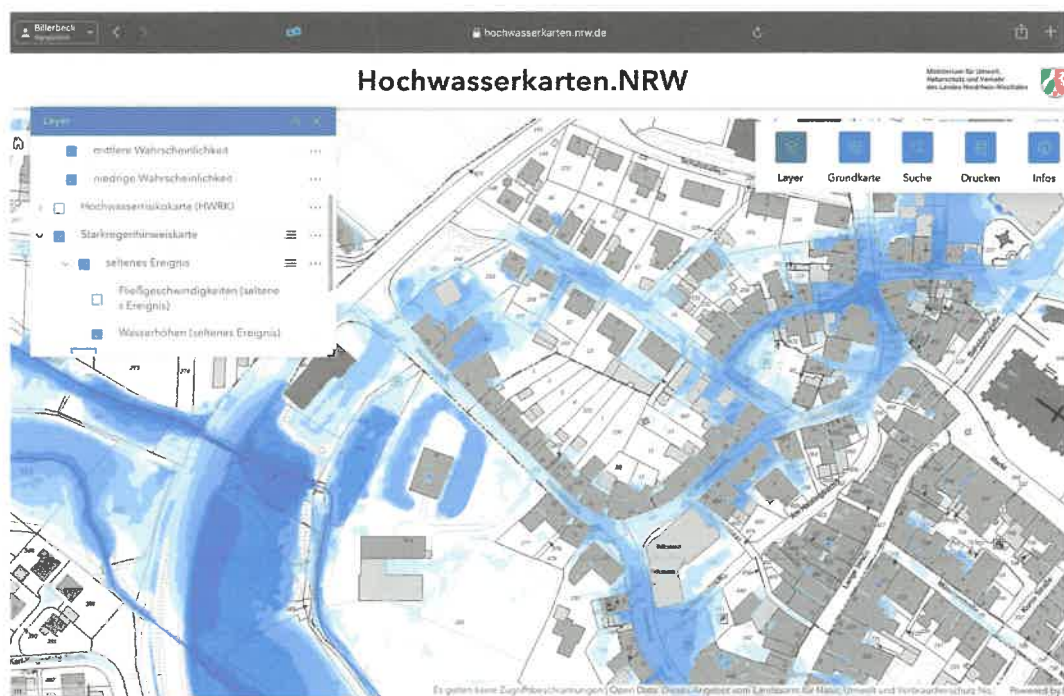
Seltenes Starkregenereignis: Wasserhöhen
